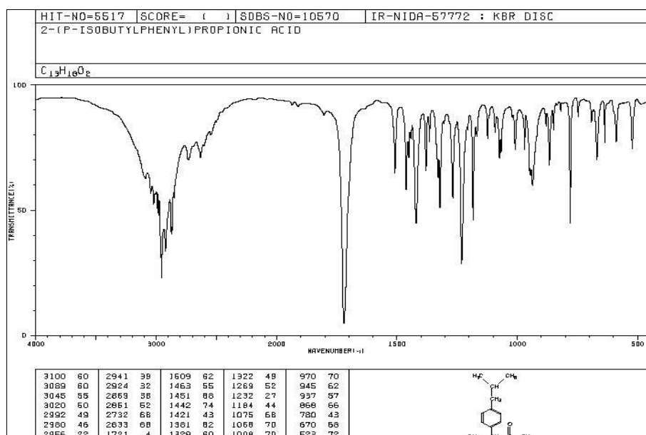
Fig 2: Spectrul ibuprofenului
